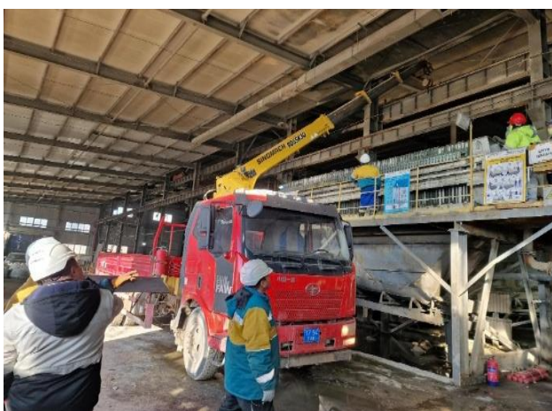
Аюулыг устгах ажил хийгдэж байна. Ачаалал даахгүй нумарч эргэсэн С төмөр болон нэмэлтээр хажууд нь хийсэн С төмрийн харагдах байдал
